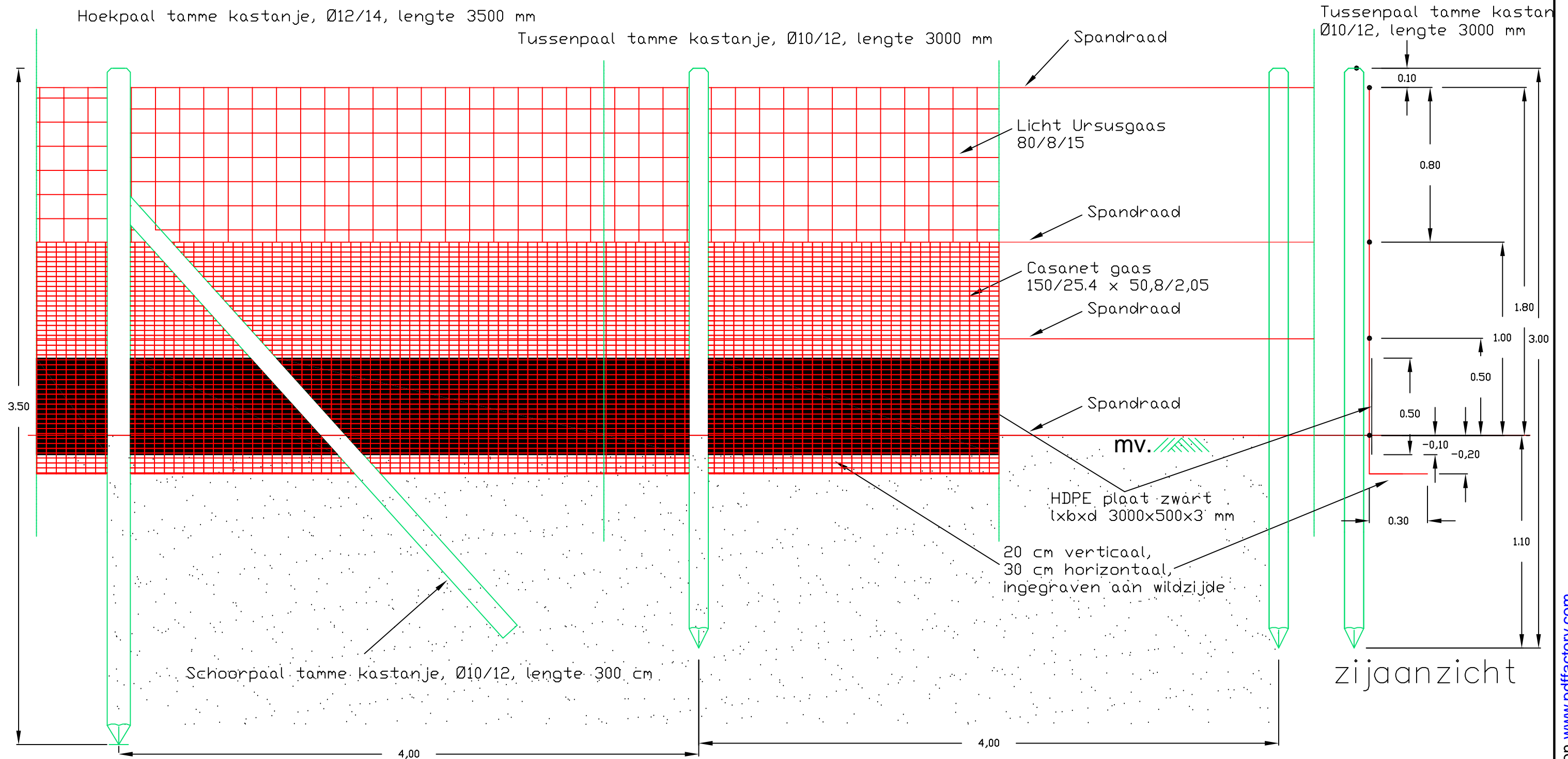
Vooraanzicht
